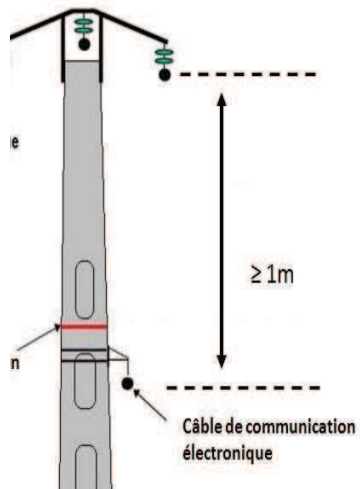
Réseau HTA nu
